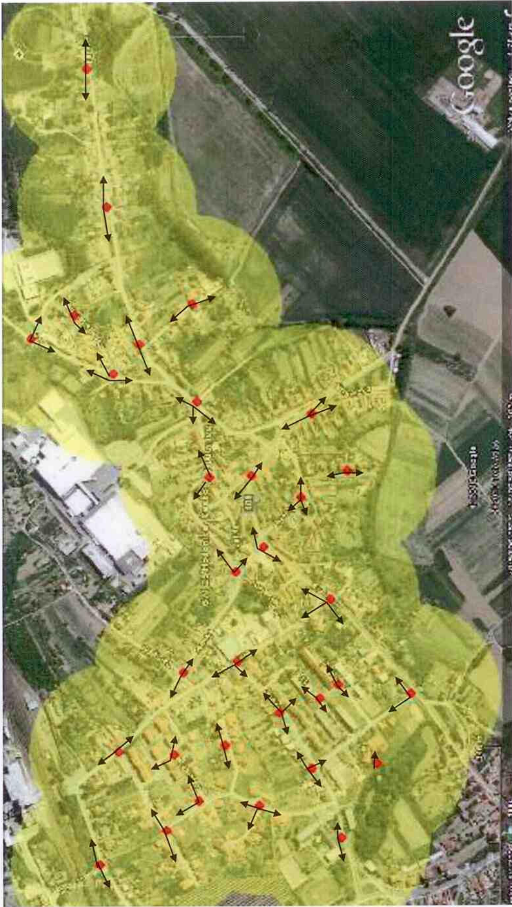
Návrh rozmístění venkovních přijímačů, reproduktorů a jejich akustický dosah v obci Hodonice
