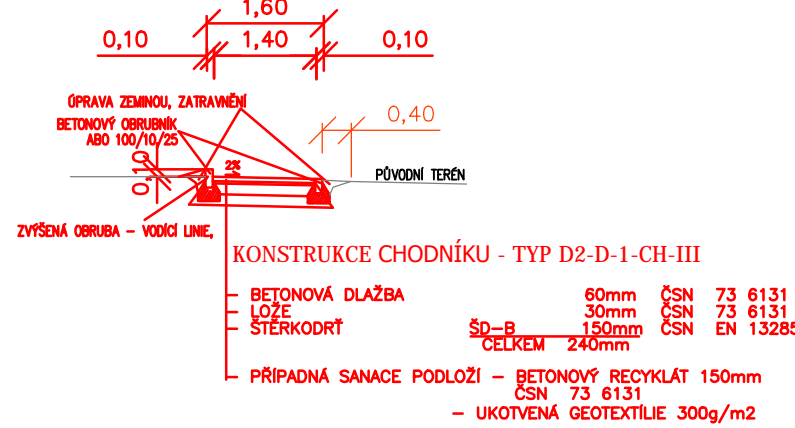
VZOROVÝ ŘEZ CHODNÍKU S OBOUSTRANNOU OBRUBOU A VODICÍ LINIÍ m.1:100
