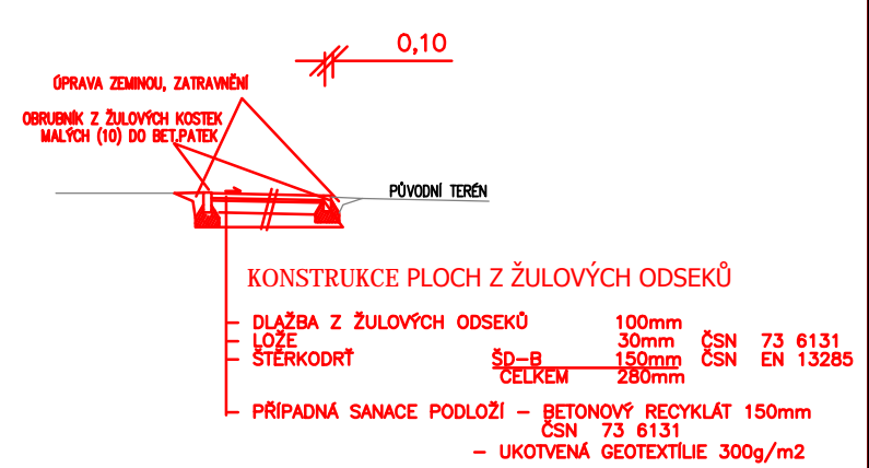
ŘEZ PLOCH Z ŽULOVÝCH ODSEKŮ m.1:100
